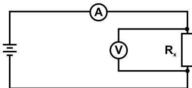
Medición de resistencia con el método técnico (sistema con la tensión correctamente medida)
