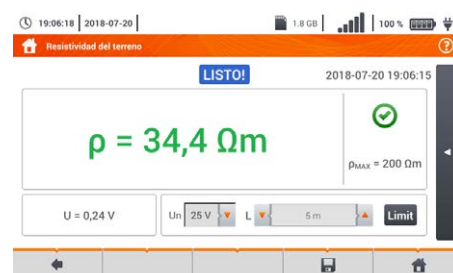
Medición de la resistividad del suelo
