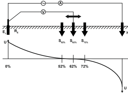
Distribución de la tensión durante el flujo de la corriente de medición
